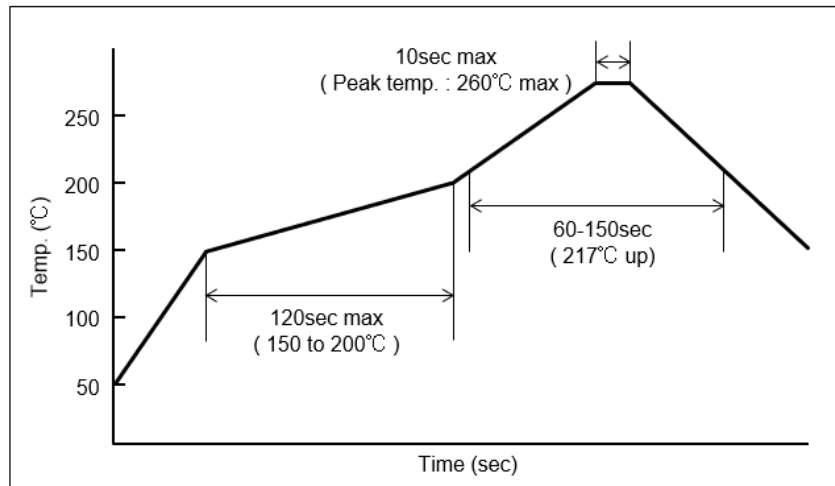
＜図-1＞ 弊社推奨リフロープロファイル ピーク温度：260℃まで
