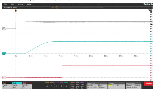
EN Start-up (Vin=12V, Vout=5.0V, Iout=10A, Cout=400uF)
