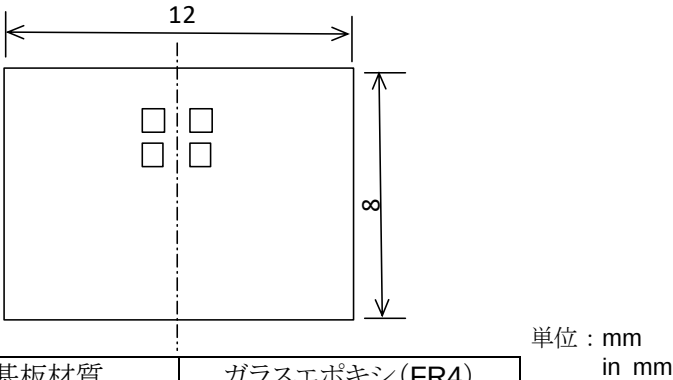
第5図 たわみ試験用基板 Figure 5. Test Board for Bending Strength Test
