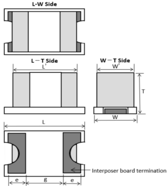
図:寸法
