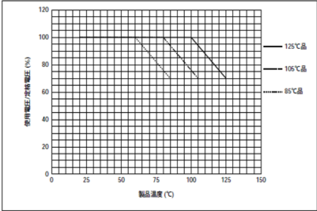
電圧・温度軽減(ディレーティング)条件 (定格電圧100V以下品)
