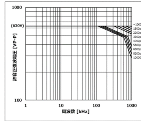
チップ(L×W):3.2×1.6mm COG(5C)特性、定格電圧:DC630V
