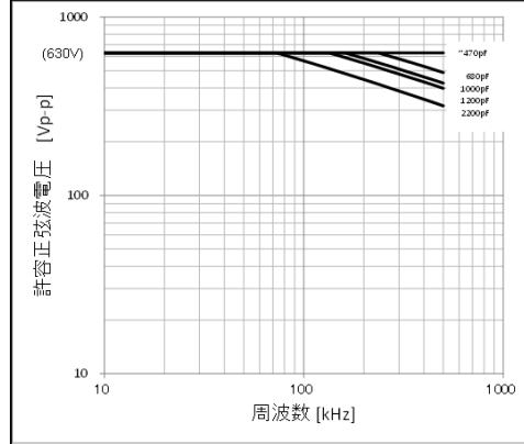
チップ(L×W):2.0×1.25mm COG(5C) 特性、定格電圧:DC630V
