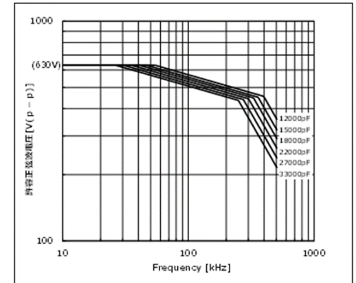
チップ(L×W):3.2×2.5mm COG(5C)特性、定格電圧:DC630V
