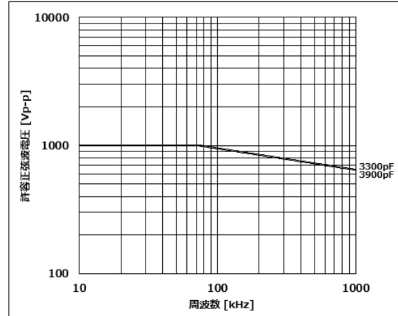
チップ(L×W):3.2×1.6mm COG(5C) 特性、定格電圧:DC1kV 静電容量範囲:3300pF to 3900pF
