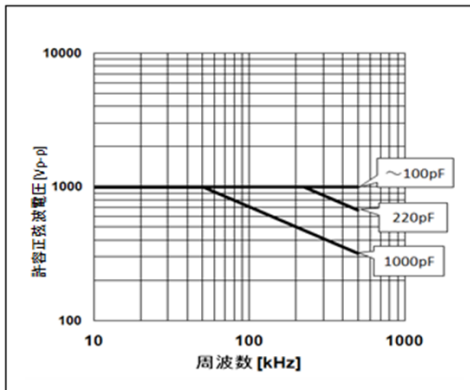
チップ(L×W):3.2×1.6mm COG(5C)特性、定格電圧:DC1kV 静電容量範囲:1000pF以下
