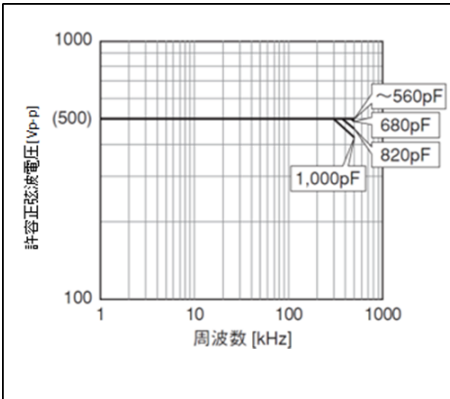
チップ(L×W):3.2×1.6mm COG(5C)特性、定格電圧:DC500V
