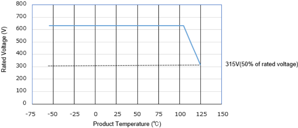
Fig:Dyrating
