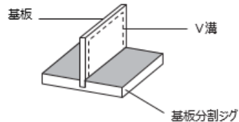
〔ジグ概要〕
