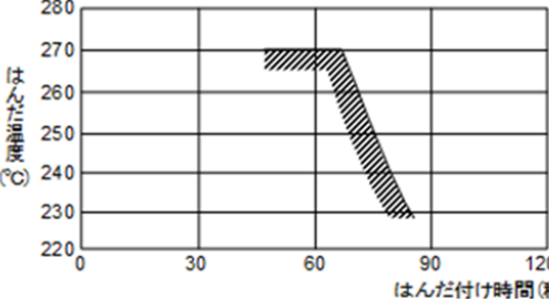
[ リフローはんだ付け許容温度、時間 ]
