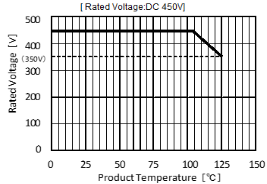
Fig:Dyrating
